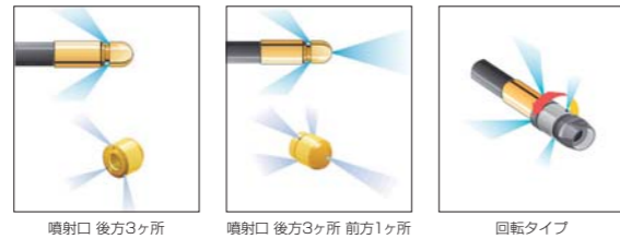
パイプクリーニングホース ノズルの種類
