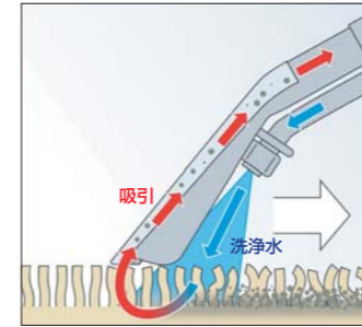
カーペットリンスクリーナーイメージ 洗剤を吹き付け、パキュム機能で吸い取ります。
